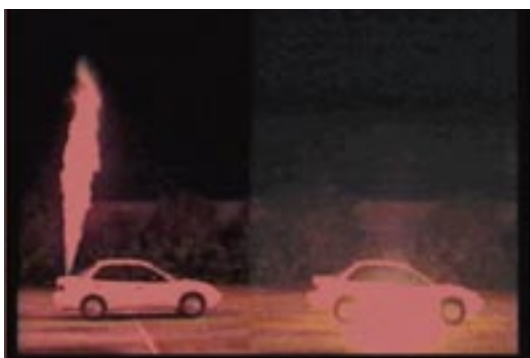
Figuur 15: Vergelijking van een brand met waterstof (wagen links) en benzine (wagen rechts). Foto links: 3 seconden na ontsteking; foto rechts: 60 seconden na ontsteking (Bron: Swain, 2001).
