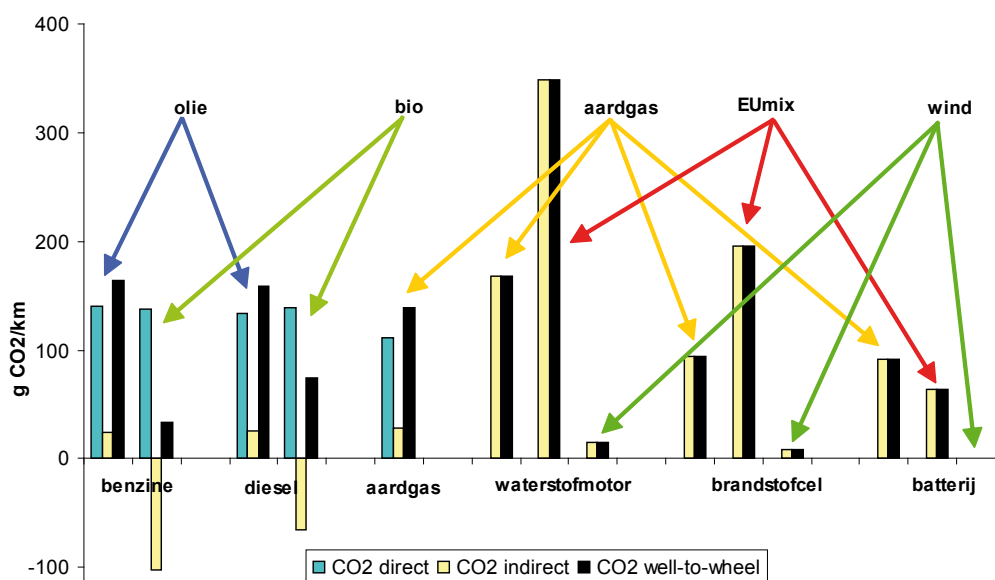
Figuur 14: Well-to-wheel CO 2 -emissies (zwart) van personenvoertuigen met verschillende brandstoffen (weergegeven bovenaan) en aandrijflijnen (weergegeven onderaan), opgedeeld in directe (blauw) en indirecte (geel) emissies.
