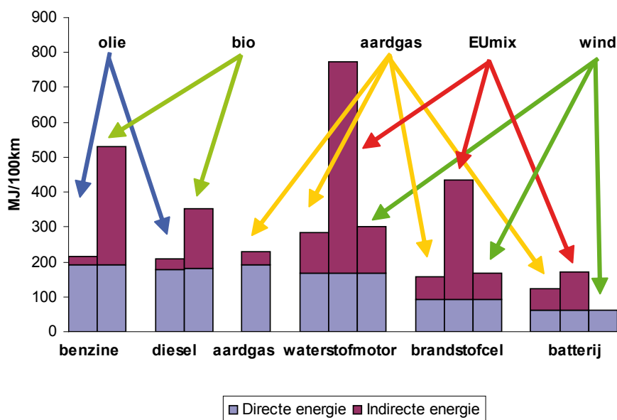
Figuur 13: Projectie van het well-to-wheel energiegebruik van personenvoertuigen met verschillende energiedragers en aandrijflijnen in 2010, opgesplitst in direct (tank-to-wheel of TTW) en indirect (well-to-tank of WTT) energiegebruik. De verschillende energiedragers zijn bovenaan weergegeven, de mogelijke aandrijflijnen onderaan.
