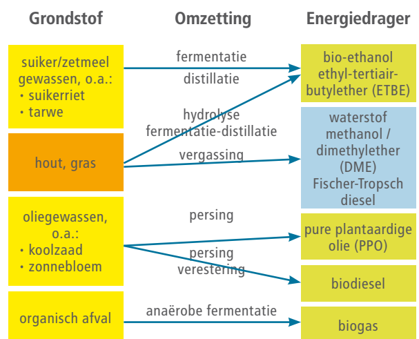
Figuur 6: Overzicht van de verschillende biobrandstoffen en hun productiepaden (eerste generatie biobrandstoffen weergegeven in geel/groen, tweede generatie in oranje/blauw).
